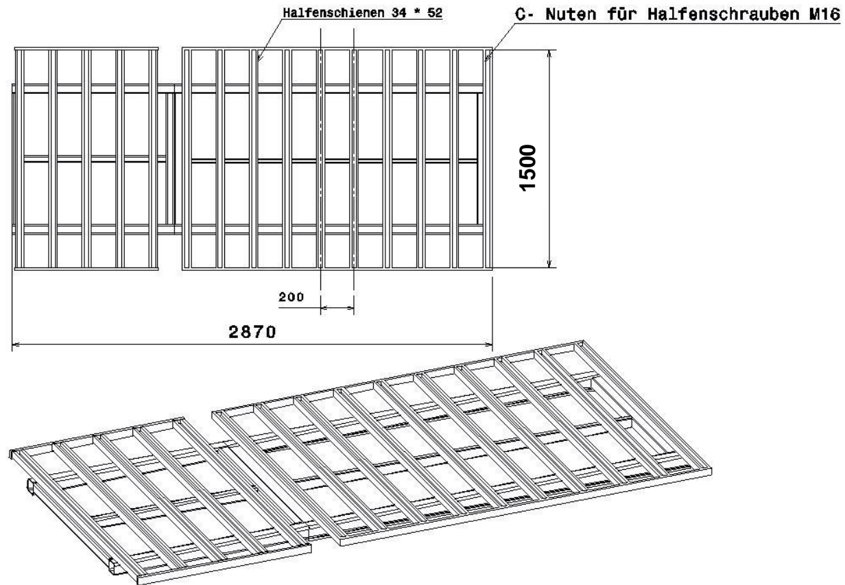
Prüfslitten mit Halfen- Adaptionstruktur, Draufsicht
